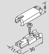
Zijgeleidsbeugel voor onderzijde montage (optioneel)
