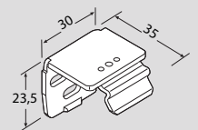
Beugel voor achterzijde montage
